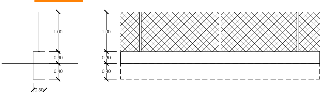
CIERRE PARCELAS, E:1/50
